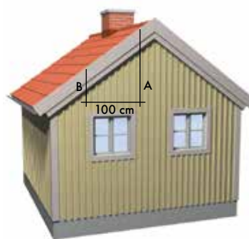
2 pav. Norėdami apskaičiuoti stogo nuolydį atimkite skaičių (B) iš skaičiaus (A) (žr. 1 lentelė)
