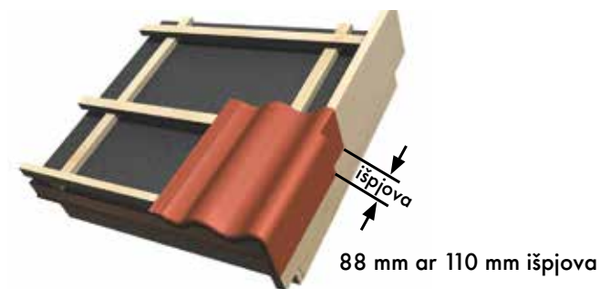
20 pav. Vietovėse kur galimi stiprūs vėjai, patariama naudoti Originalias kraštines (dešininės/kairinės) čerpes.
