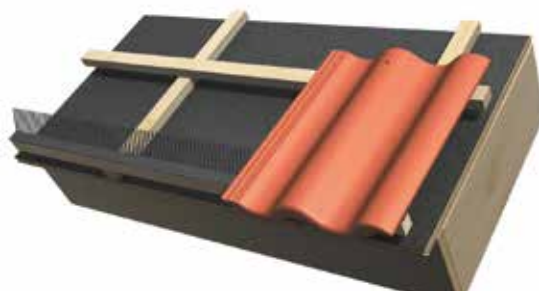
27 pav. Apsauga nuo paukščių pritvirtinama ant apatinio karnizo grebėsto. Taip neleidžiama paukščiams susukti lizdų po čerpėmis. Siūlomos skirtingos apsaugos – su ventiliacija ir be jos.
