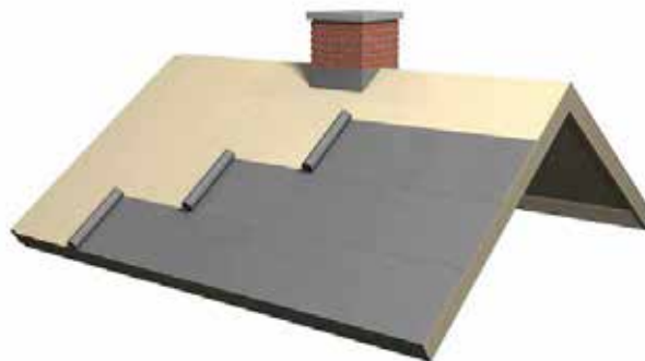
3 pav. Stogo plėvelė pradama kloti nuo stogo apačios(karnizo) iki kraigo horizontalia kryptimi ir tvirtinama ventiliaciniais tašeliais.
