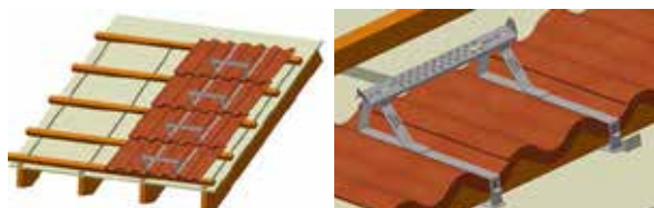
33 pav. Stogo kopetėlės montuojamos ant to paties grebėsto kaip ir stogo čerpės, užkabinant ją už grebėsto.
